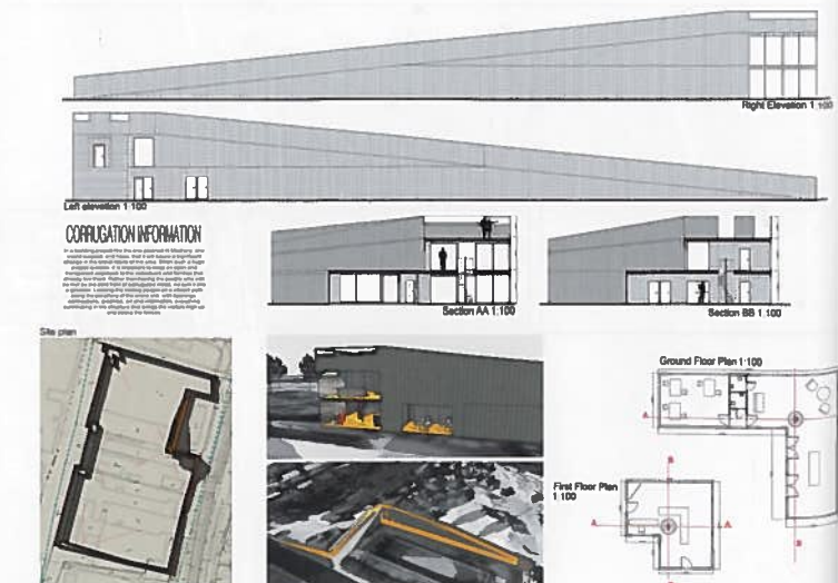
Práce Architectural Design 1, autor: Feliks Isaksen (Loukotová studio)
